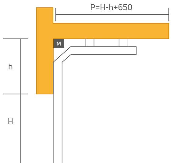
Architrave parzialmente verticale
