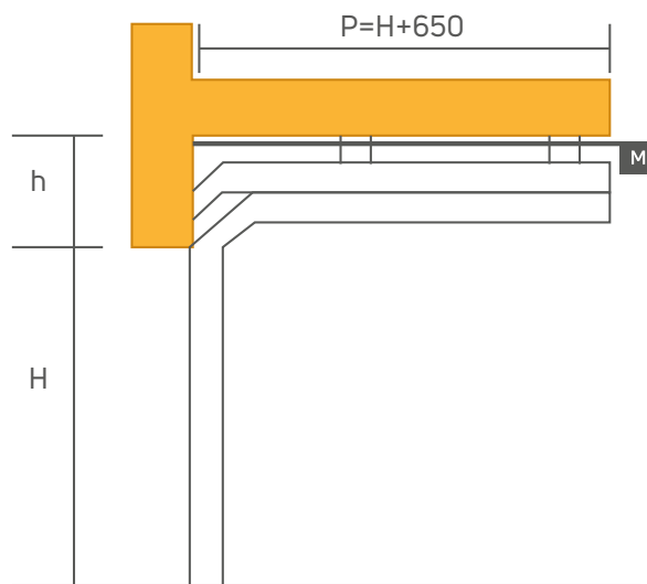
Architrave ribassato
